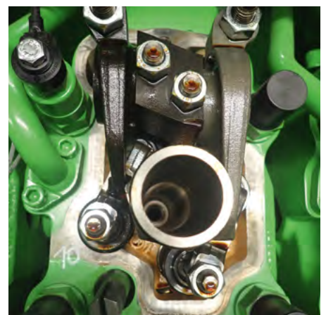
Головка цилиндра с клапанным механизмом INNIO Jenbacher J416 GS-B02
