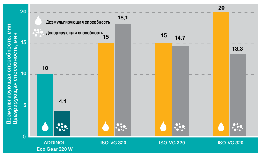
График 3. Деземულიрующая и деаэрирующая способность синтетических трансмиссионных масел согласно стандартам DIN ISO 6614 (82 °C), DIN ISO 9120 (75 °C)
