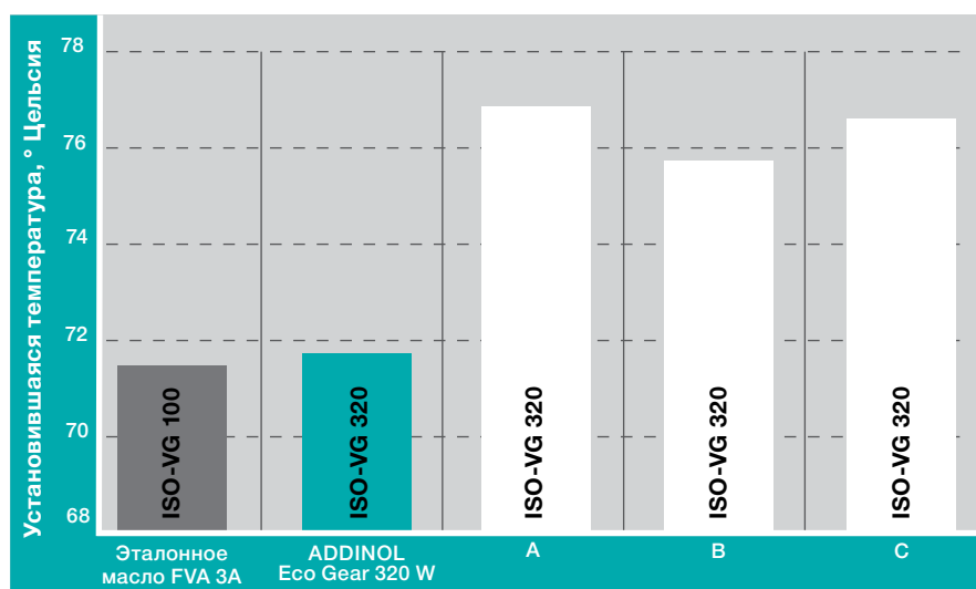
График 1. Сравнение показателей установившейся температуры синтетических трансмиссионных масел ISO VG 320 по методу FVA 345* на 7 ступени нагрузки
