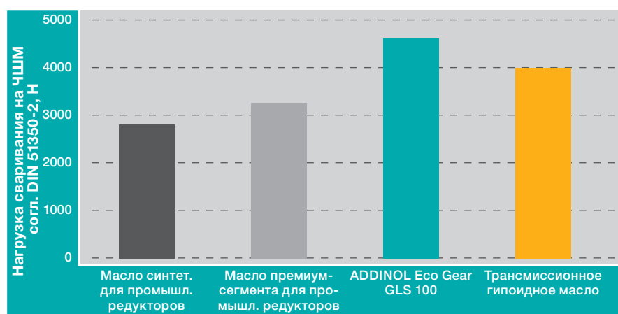
График 5. Несущая способность синтетических трансмиссионных масел
